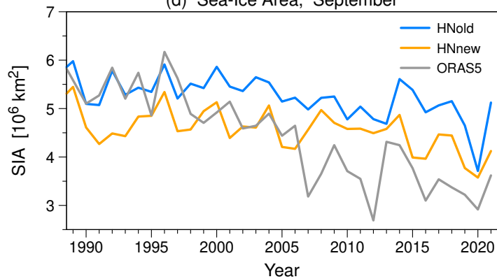
(d) Sea-Ice Area, September
